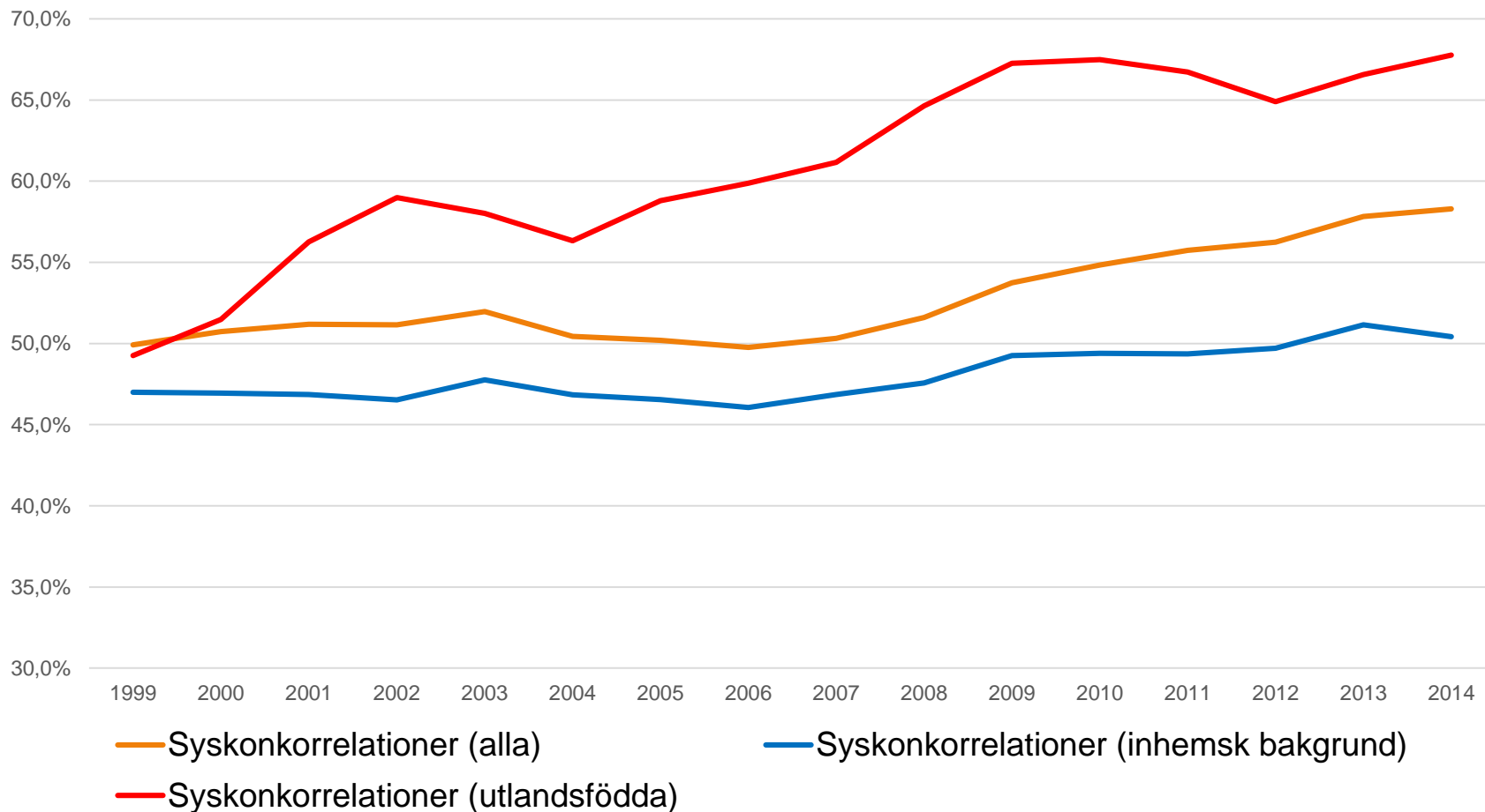
Syskonkorrelationer (betyg i matematik och engelska)
